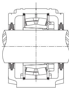
VEDAÇÃO TG C/ DUPLO RASPADOR
