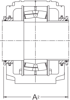
VEDAÇÃO TS ANÉIS DE LABIRINTO
