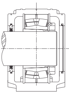
VEDAÇÃO TC e VEDADORES DE FELTRO
